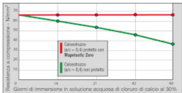
Fig.4: Effetto Mapelastik Zero sul decadimento meccanico del calcestruzzo dovuto ai sali disgelanti a base di cloruro di calcio
