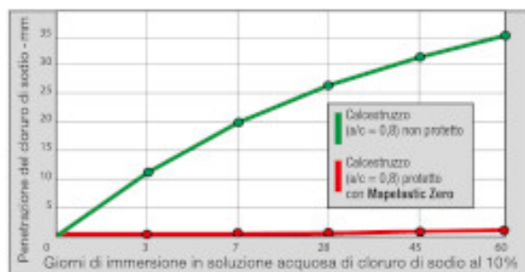
Fig.3: Effetto Mapelastik Zero sulla penetrazione del cloruro di sodio in un calcestruzzo poroso
