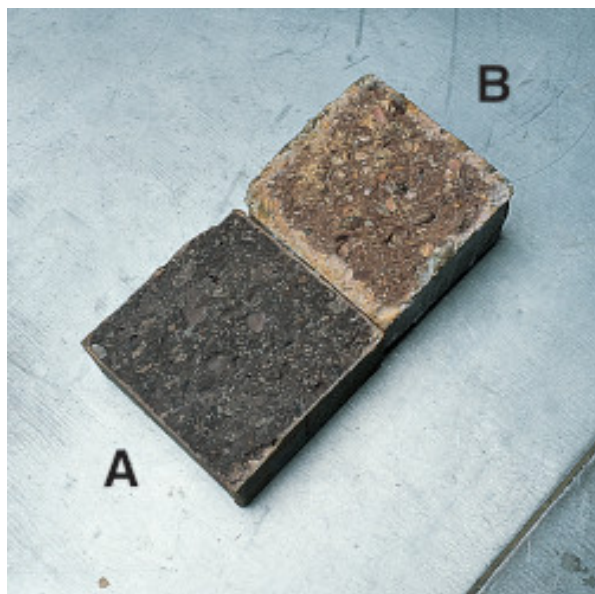
Fig. 2 B - Prove di penetrazione dello ione cloruro (UNI 9944). Il campione A, rivestito con Mapelastik Zero , risulta non penetrato; il campione B, tal quale, presenta un fronte di avanzamento di diversi millimetri
