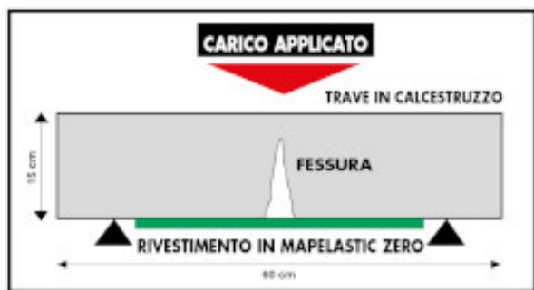
Fig.1: Protezione con Mapelastik Zero di una fessura all'intradosso di una trave in calcestruzzo sottoposta a una sollecitazione flessionale
